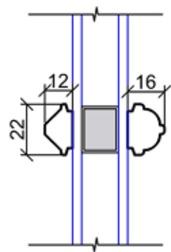
Glazing Bar
