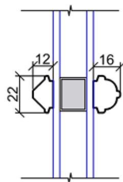
Glazing Bar
